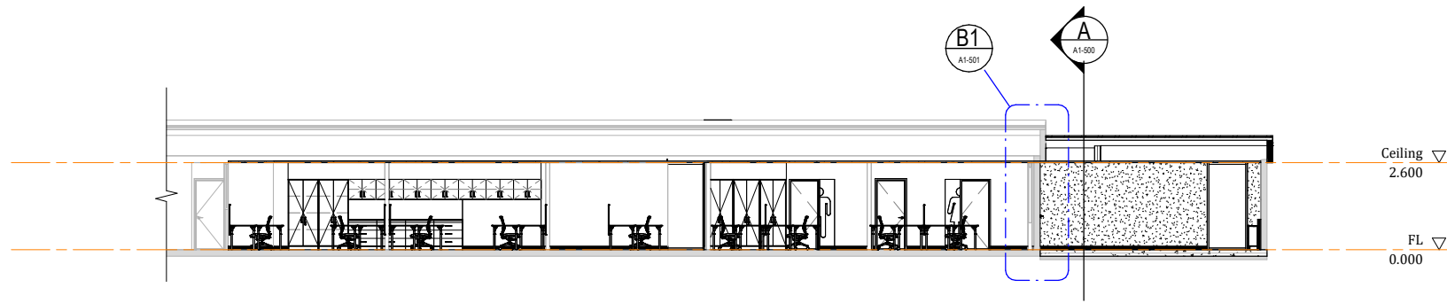
Section B 1 : 100
