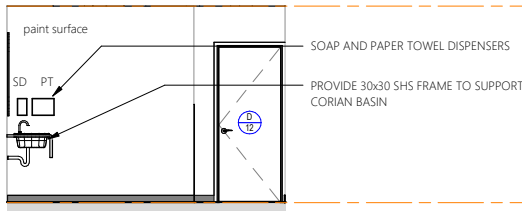
Elevation 4B
