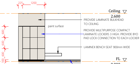
Elevation 4G
