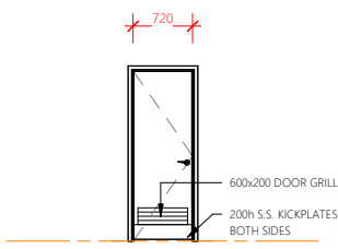
DOOR TYPE D
