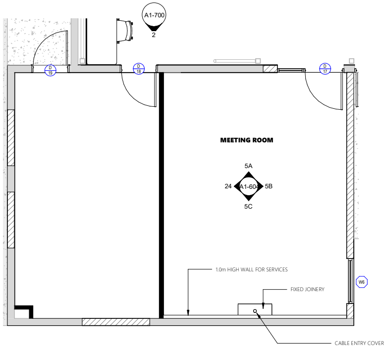
Internal Plan 5 1 : 50
