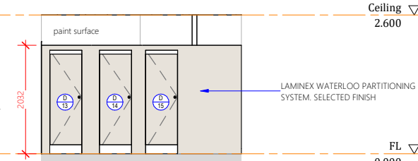
Elevation 4E
