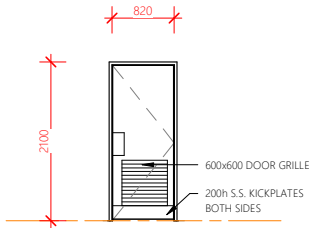
DOOR TYPE C
