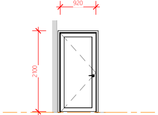
DOOR TYPE H
