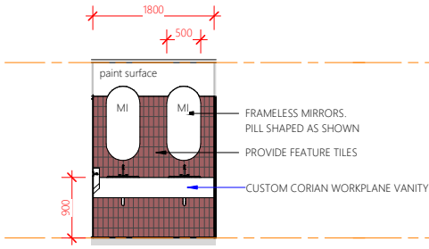
Elevation 4A
