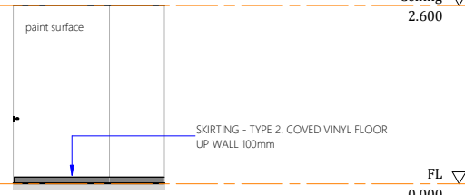
Elevation 4C
