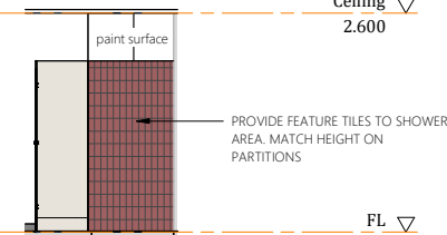
Elevation 4J
