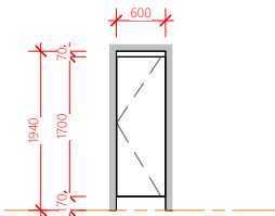
DOOR TYPE E
