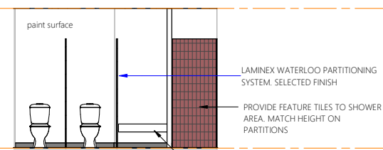
Elevation 4I
