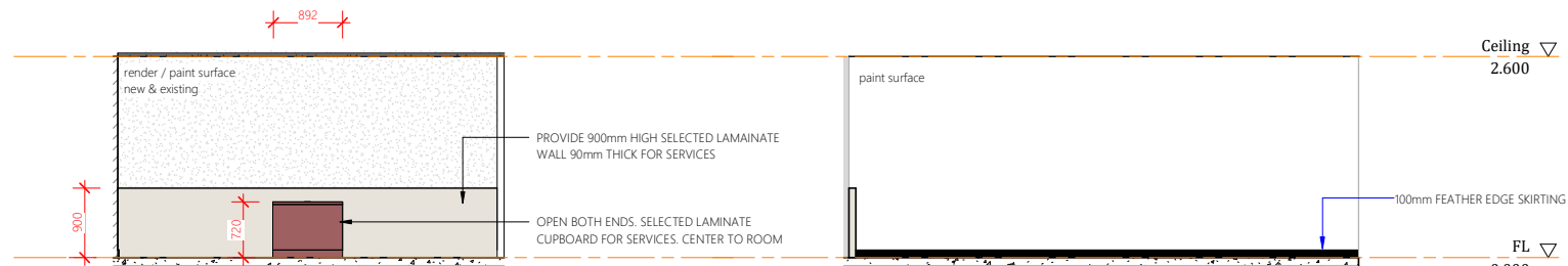
Elevation 5C 1 : 50
